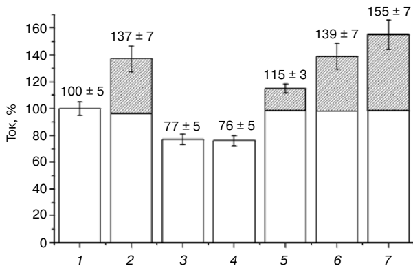
Рис. 4. Интенсивность пиков квадратно-волновых вольтамперограмм в аэробных условиях электродов: DDAB/Au/P450 3A4 (1); DDAB/Au/P450 3A4 + DF, 100 мкМ (2); DDAB/Au/P450 3A4 + ITR, 10 мкМ (3); DDAB/Au/P450 3A4 + ITR, 10 мкМ, затем DF, 100 мкМ (4); DDAB/Au/P450 3A4 + TAU, 50 мкМ (5); DDAB/Au/P450 3A4 + TAU, затем ITR (6); DDAB/Au/P450 3A4 + ET, 180 мкМ (7). Значения амплитуд токов КВВА были скорректированы по базовой линии. Приведены средние значения пяти экспериментов. TAU – таурин, ET – этоксидол
