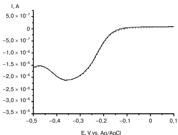
Рис. 3. Квадратно-волновые вольтамперограммы электродов: DDAB/Au/P450 3A4 + 10 мкМ ITR (сплошная кривая); DDAB/Au/P450 3A4 + 10 мкМ ITR, затем 100 мкМ DF (штрихпунктирная кривая)
